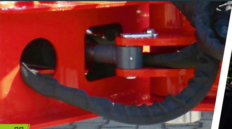
Schwenkdeichsel mit zwei geschützten Zylindern und mechanische Verriegelung für Straßenfahrten
